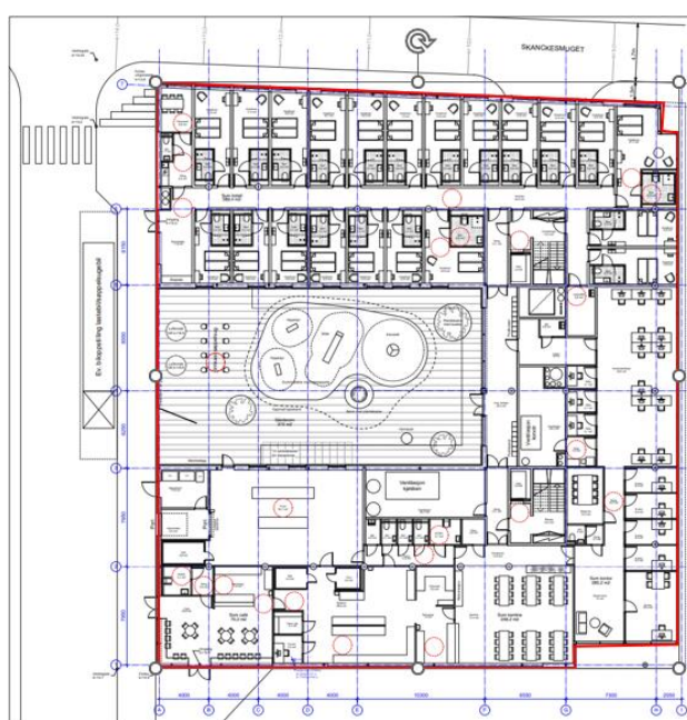
Plan 2. etasje - ASVO/hotell og kafé
