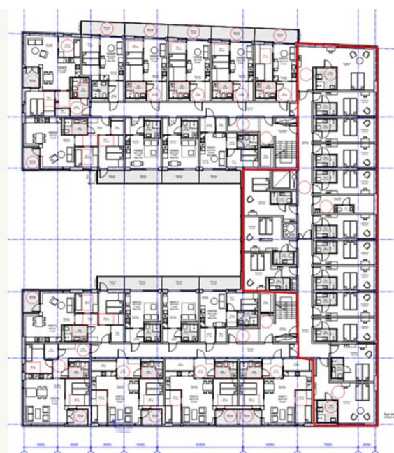
Plan 3. etasje - Bolig og ASVO/hotell
